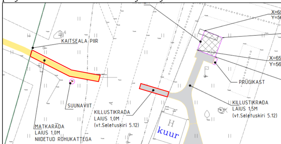
Joonis 1. Väljavõtte muuseumi parkla asendiplaanist. Riigitee alusele maale projekteeritud käiguraja ala tähistatud punase joonega.
